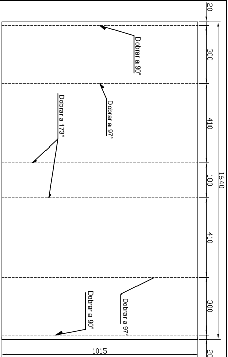
PEÇA A Chapa # 14 Quantidade: 01 Peça
